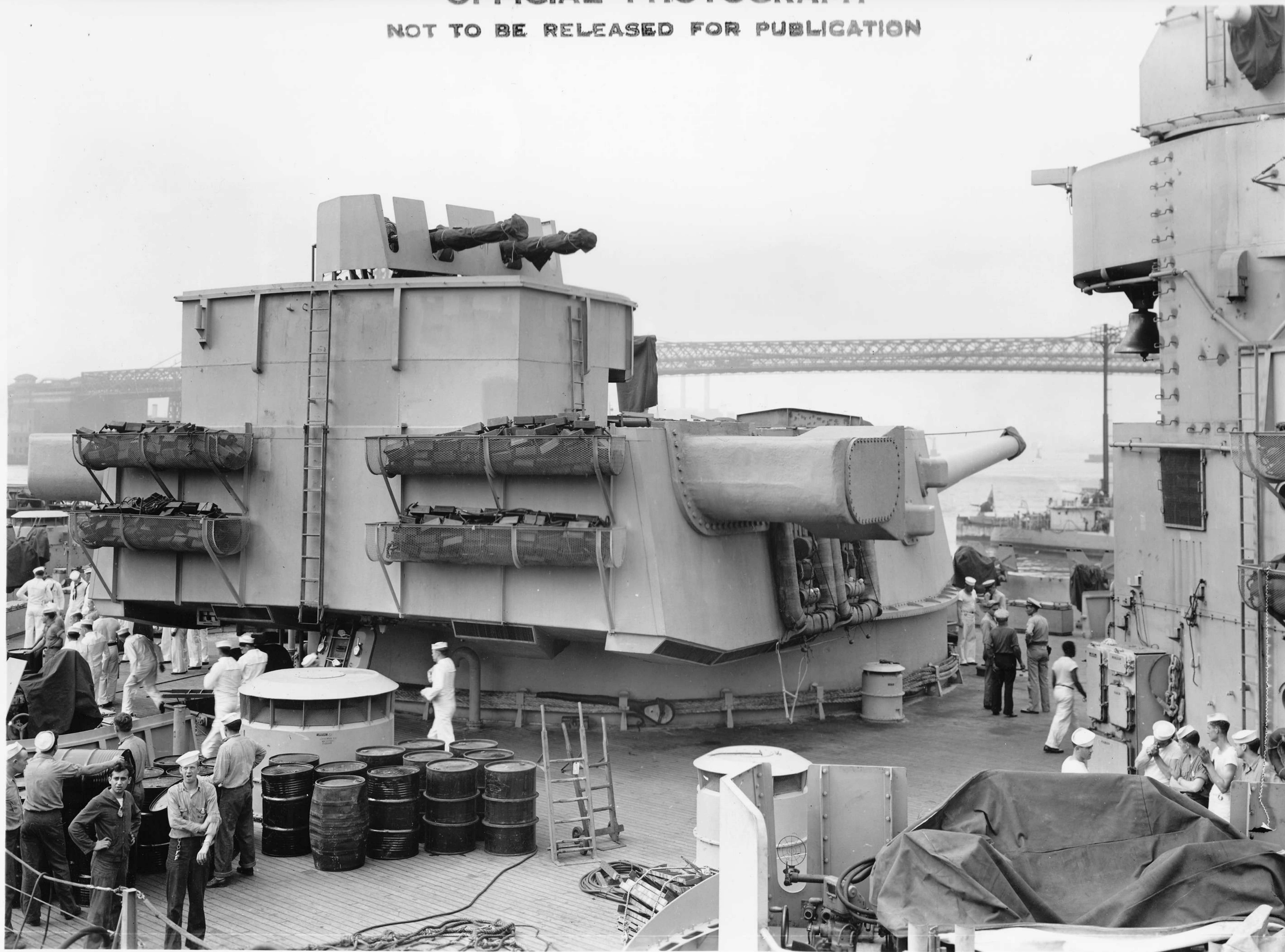
F1111C466 U. S. S. BB 61. 40 MM. MT. ON TUR. #3. SIDE VIEW.
